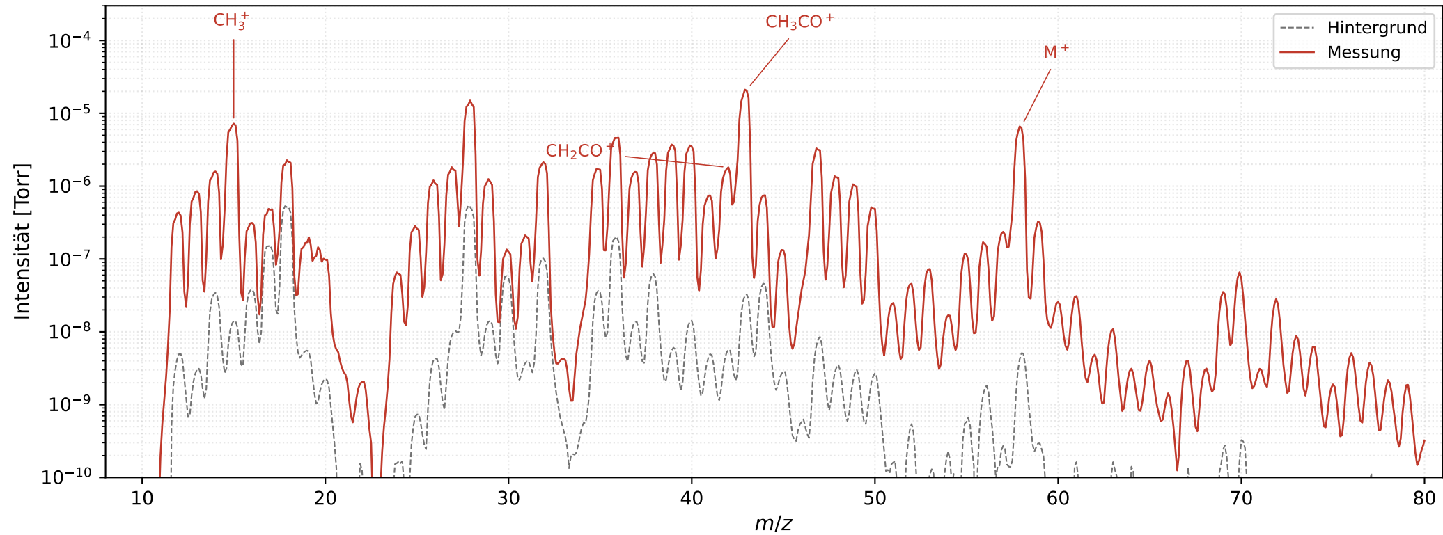
Aceton ( \text{C}_3\text{H}_6\text{O} , M = 58 ) — Messung und Hintergrund (logarithmisch)
